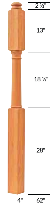
S-4246 Landing Newel
